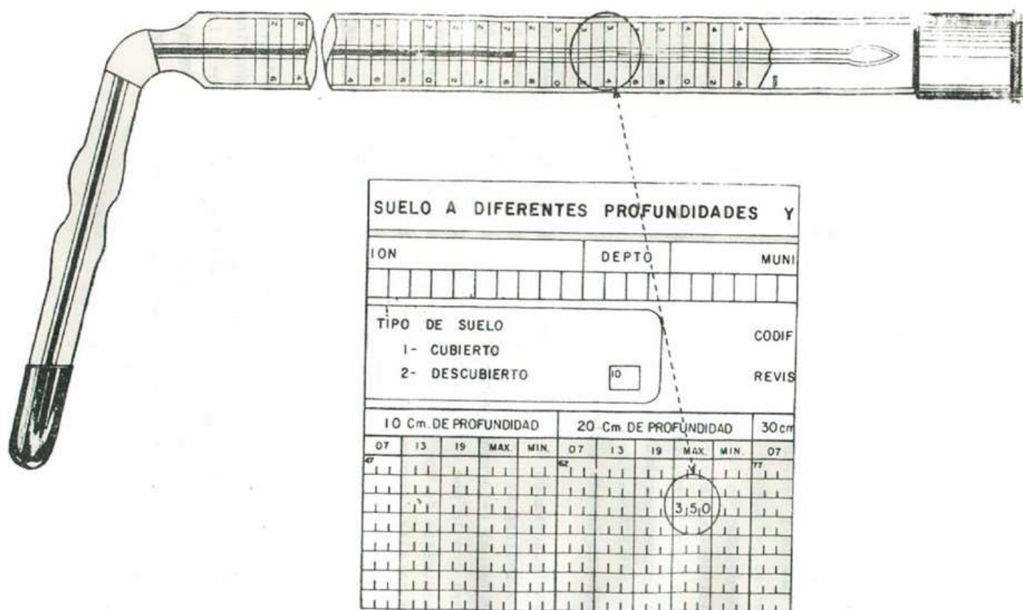
Figura 14. Geotermómetro de máxima (20cm) lectura anotada al formato
