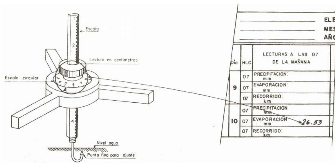
Figura 25. Tornillo micrométrico con gancho
