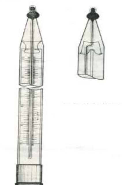
Figura 8. Termómetro de máxima con estrangulamiento
