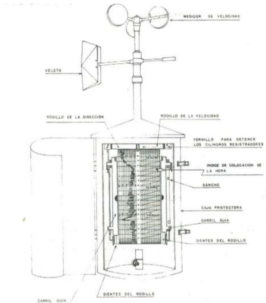
Figura 30. Anemógrafo mecánico tipo Woelfle
