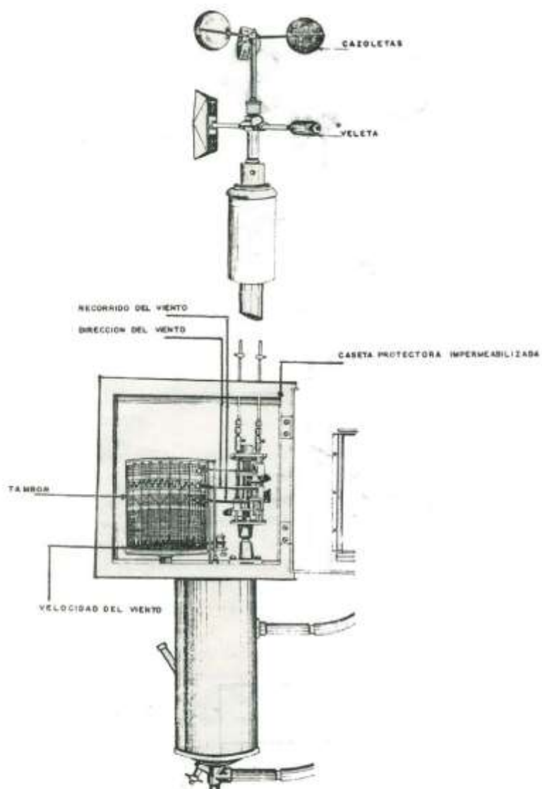
Anemógrafo
