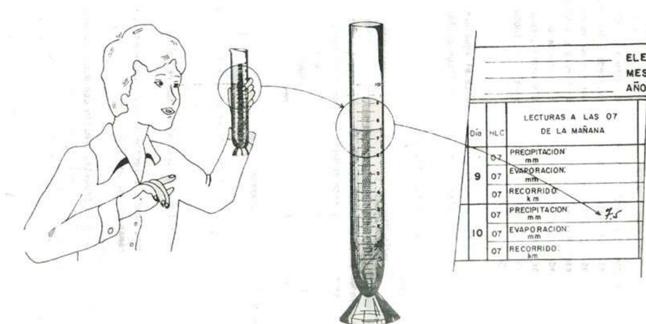
Figura 23. Lectura del pluviómetro con probeta y anotación en la libreta
