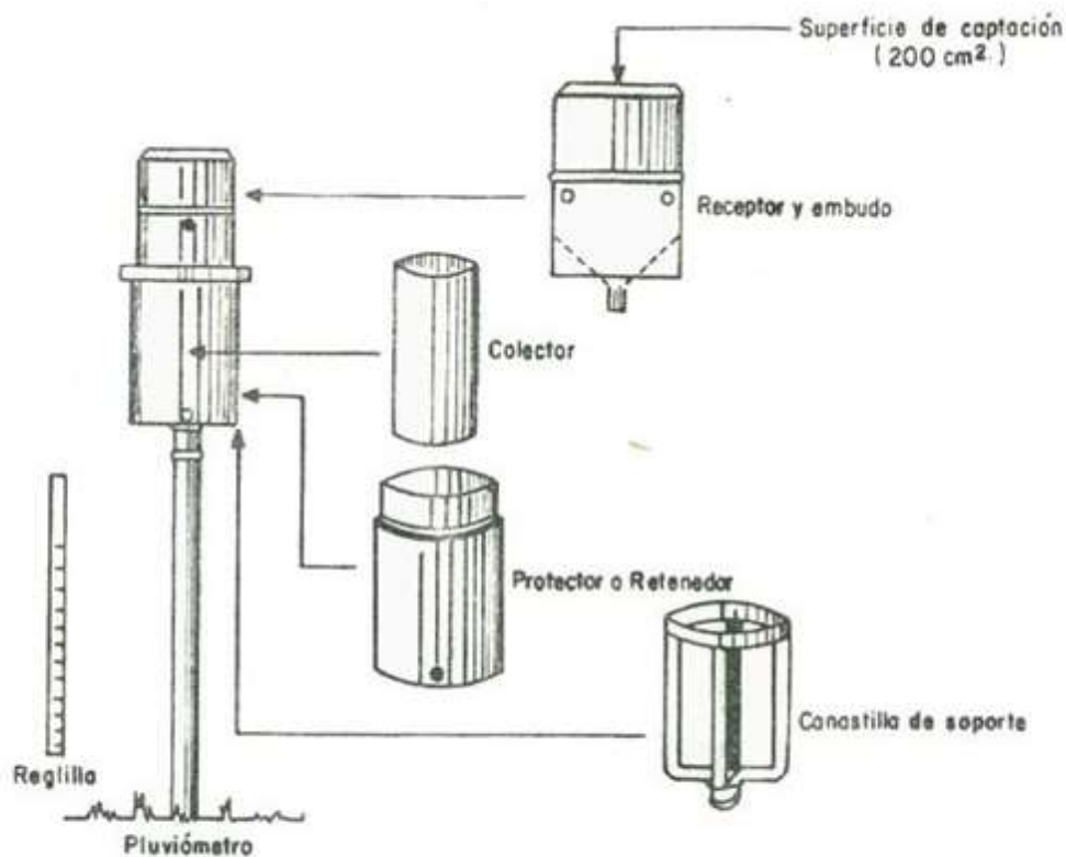
Figura 21. Elementos del pluviómetro
