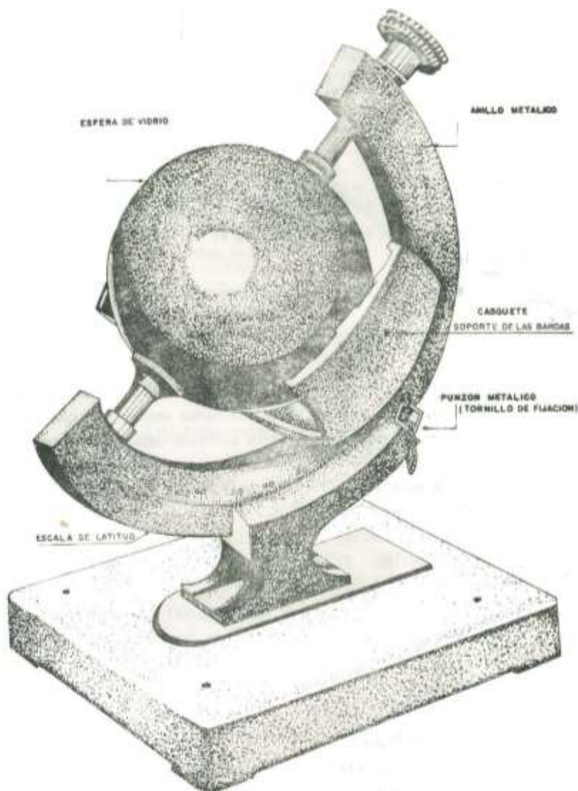
Heliógrafo
